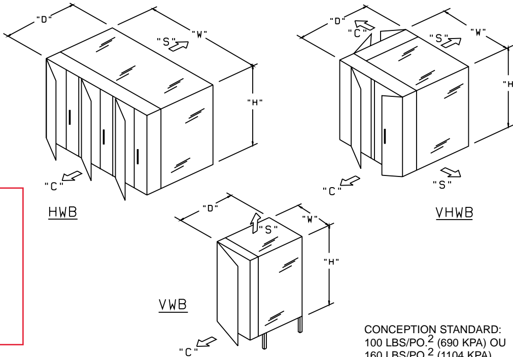
TABEAU 1 - CHAUDIÈRE À EAU CHAUDE SPÉCIFICATIONS GÉNÉRALES
