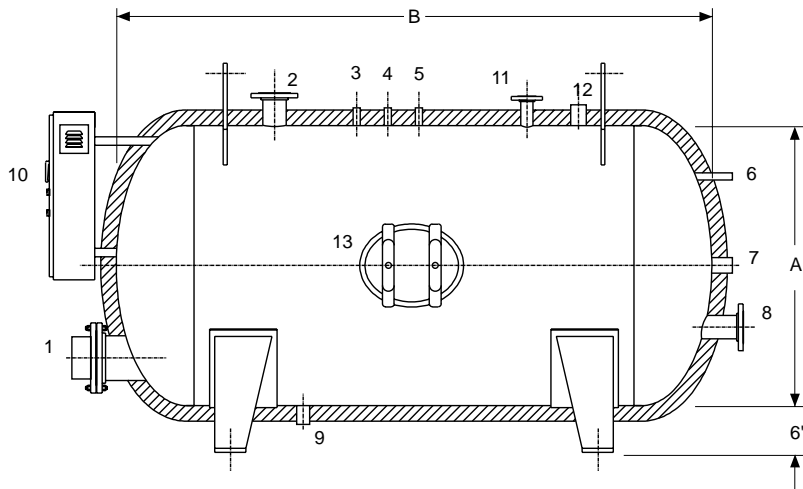
FIG. 5 - MODÈLE HC RÉSERVOIR D'EMMAGASINEMENT
