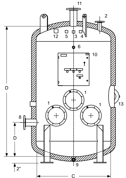
FIG. 6 - MODÈLE VC RÉSERVOIR D'EMMAGASINEMENT
